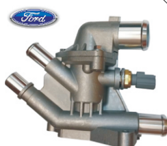
CÓD. INT. 8811 CÓD. PROD. 2015 155 VALVULA TERMOSTATICA COMPLETA NOVO KA 1.0 12V FLEX 14/...
