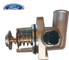
CÓD. INT. 8807 CÓD. PROD. 2015 151 VALVULA TERMOSTATICA COMPLETA FIESTA/ECOSPOT MOTOR ZETEC
