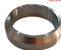
CÓD. INT. 7833 CÓD. PROD. 1500 115 ANEL ENCOSTO ROL. TRAS. HILUX PITBUL 2.8/3.0.../10 39.5X50.8X13 (15MM)
